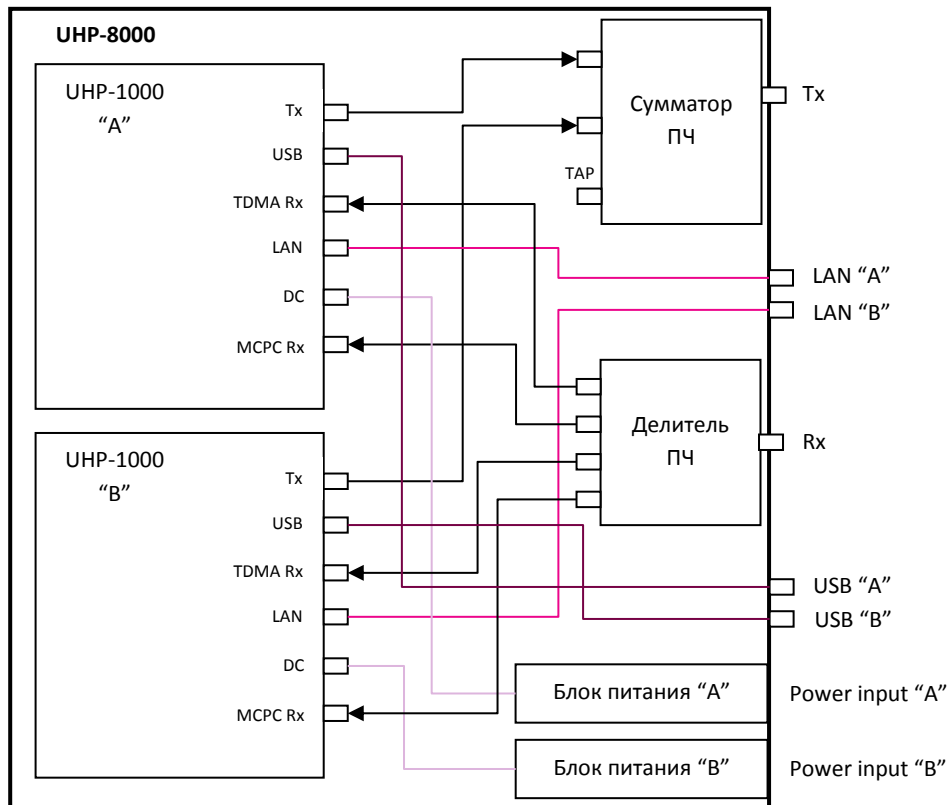
Рисунок 4 Структура маршрутизатора UHP-8000 в базовой конфигурации
