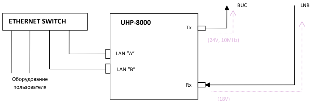
Рисунок 8 Пример подключения в базовом режиме
