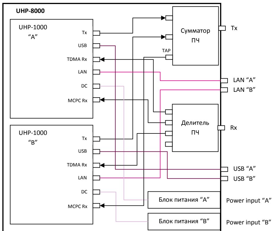
Рисунок 5 Структура маршрутизатора UHP-8000 в конфигурации HUB (HVIC)
