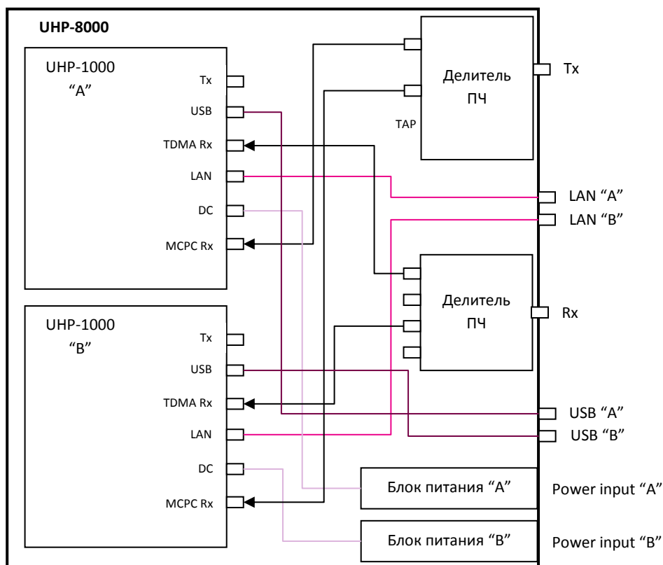
Рисунок 6 Структура маршрутизатора UHP-8000 в конфигурации ICIC
