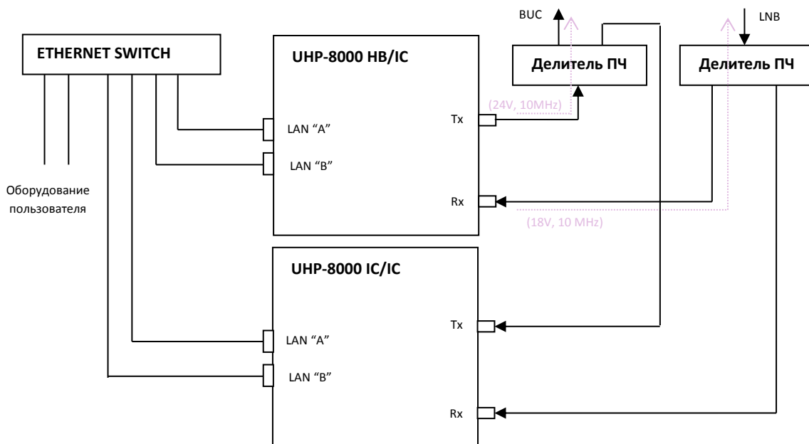
Рисунок 9 Пример подключения каскадом (Центральная станция TDM/TDMA)
